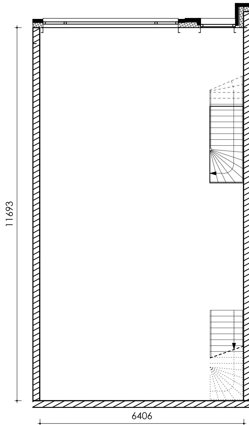
1e Verdieping
