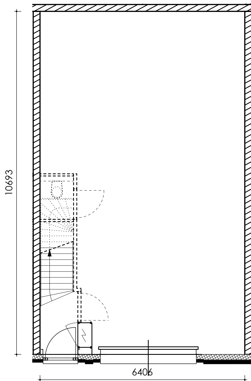
Begane Grond
