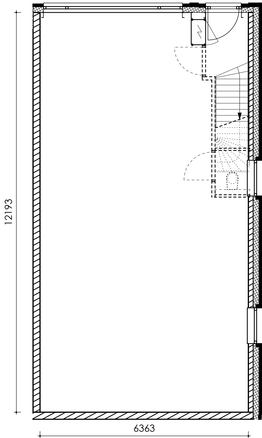
Begane Grond
