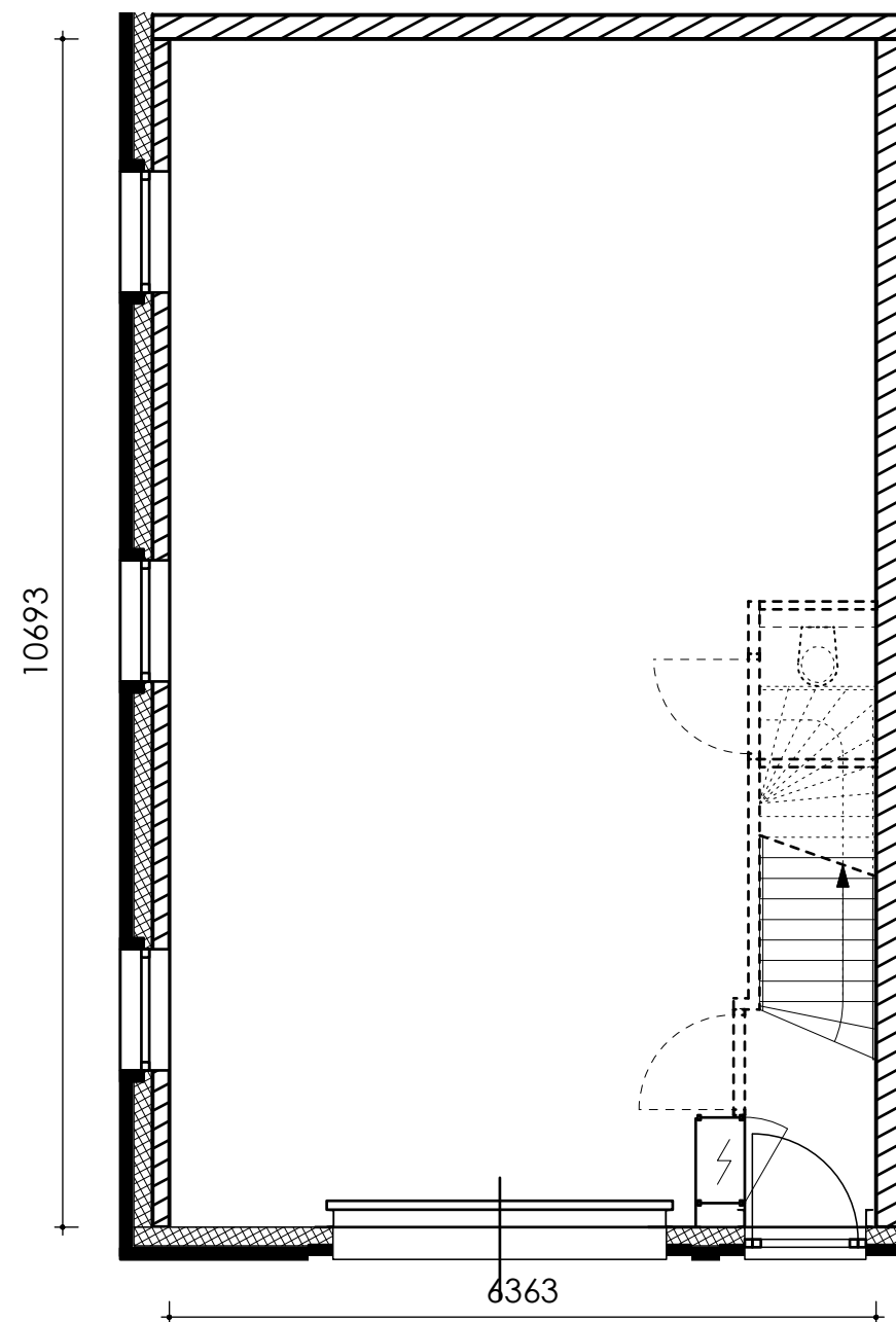
Begane Grond
