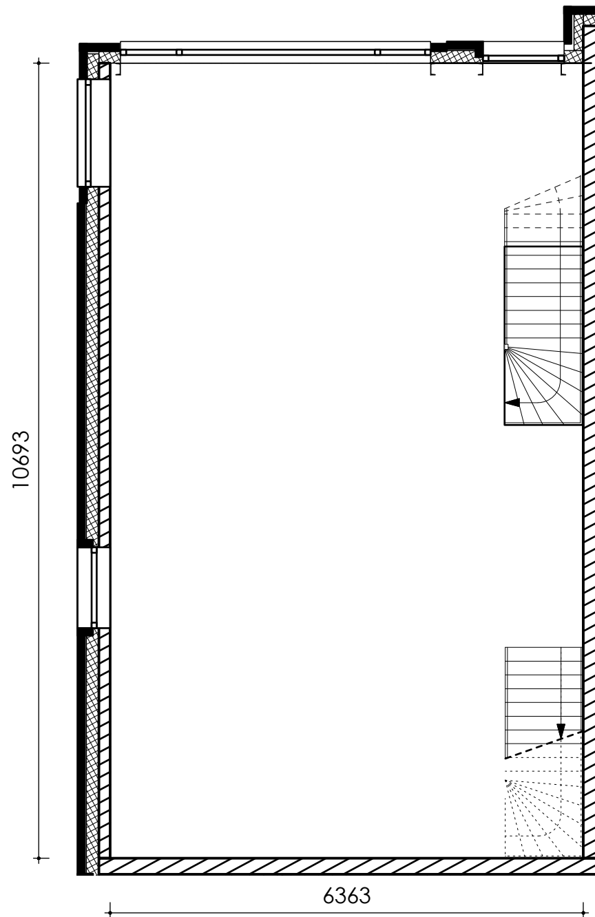
1e Verdieping
