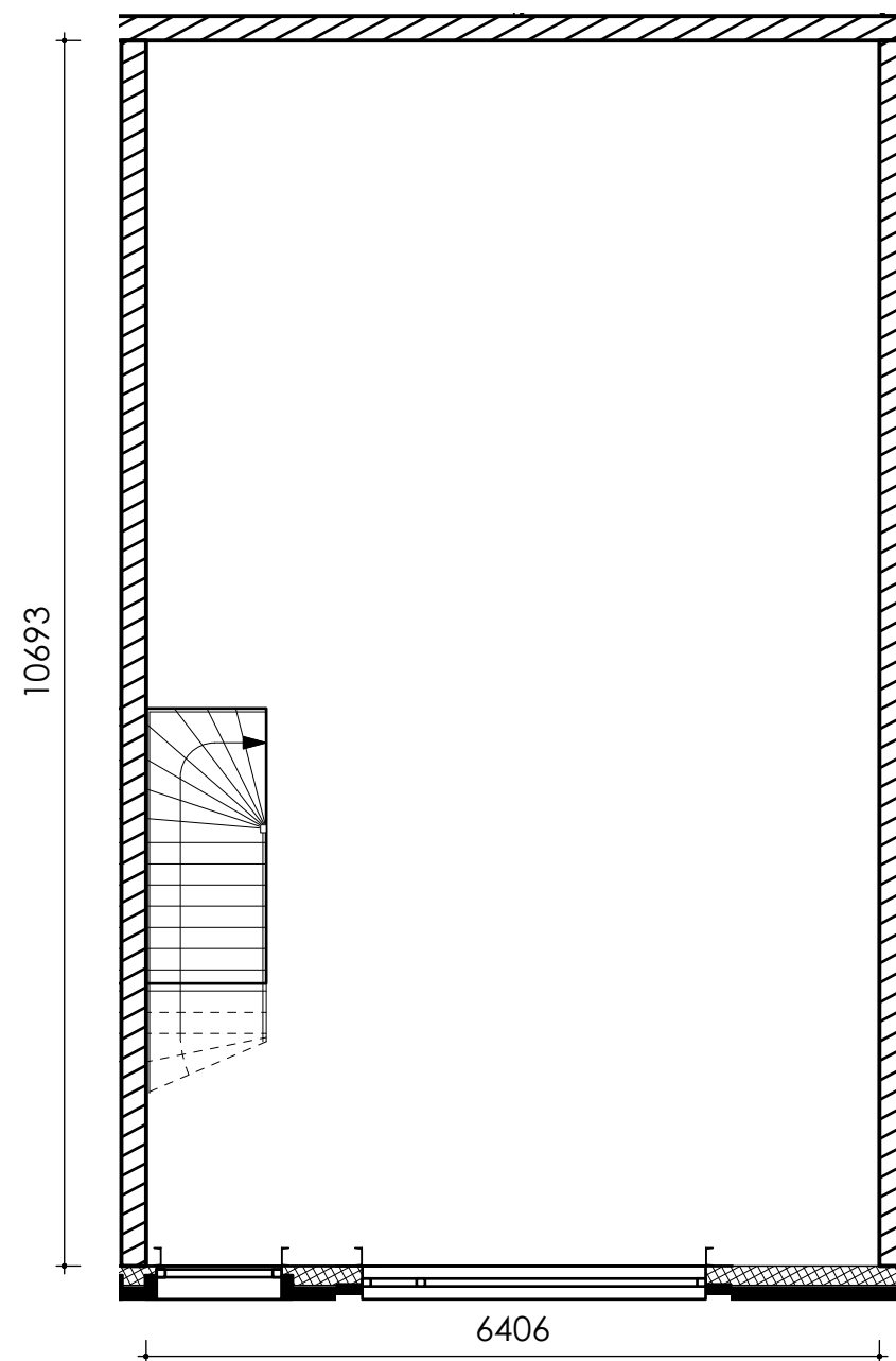
1e Verdieping
