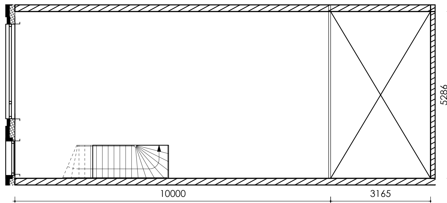
1e Verdieping
