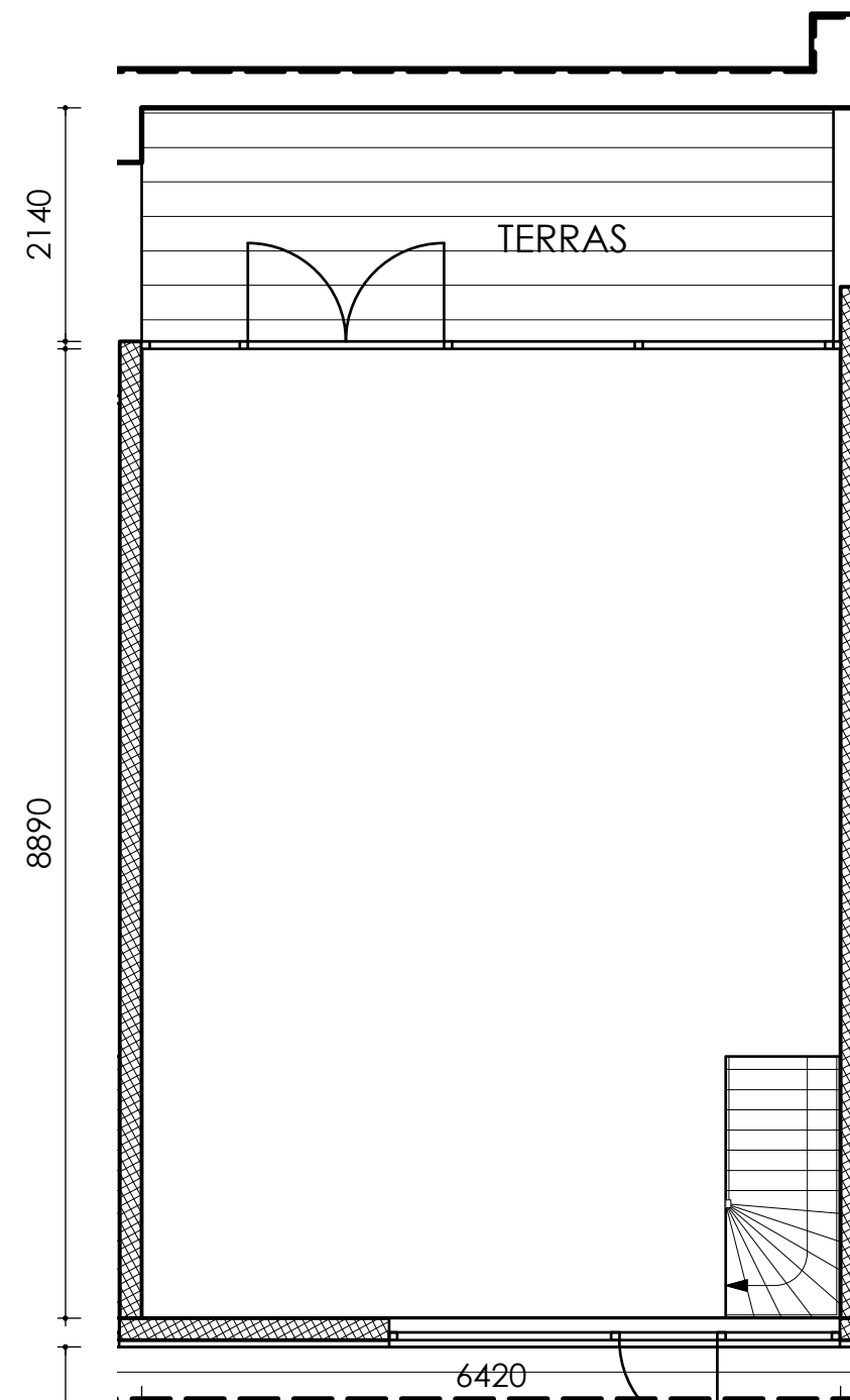
2e Verdieping
