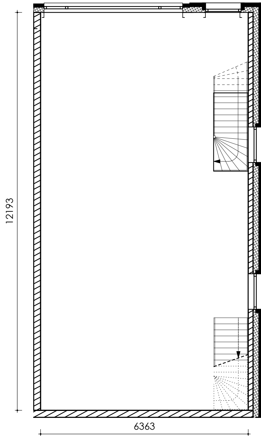
1e Verdieping
